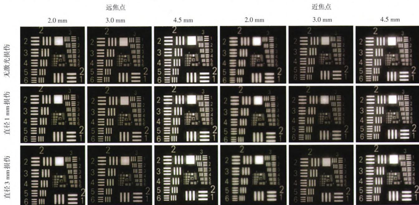
图 3 不同通光孔径下多焦点 IOL 损伤前后美军标对比图 不同损伤直径 IOL 与未损伤 IOL 远焦点美军标成像亮度无明显变化,通光直径为 4.5 mm 时 IOL 近焦点可以看到眩光现象
