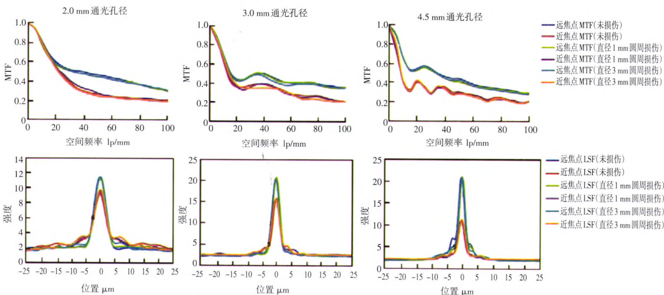
图 2 不同通光孔径下多焦点 IOL 损伤前后 MTF、LSF 曲线变化 MTF:调制传递函数;LSF:线扩散函数
